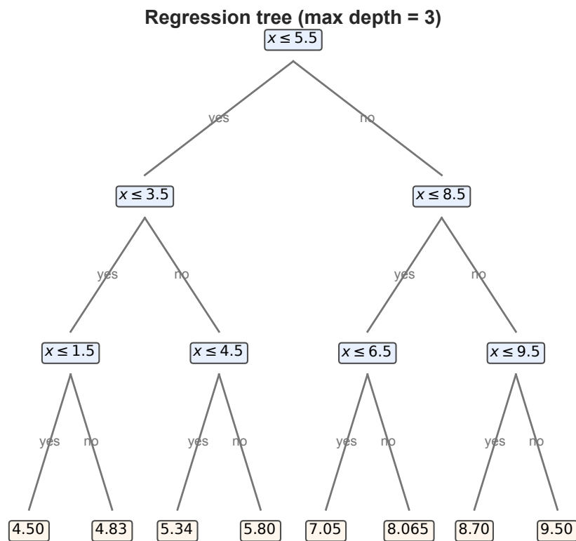
图 4: 深度为 3 的最小二乘回归树
